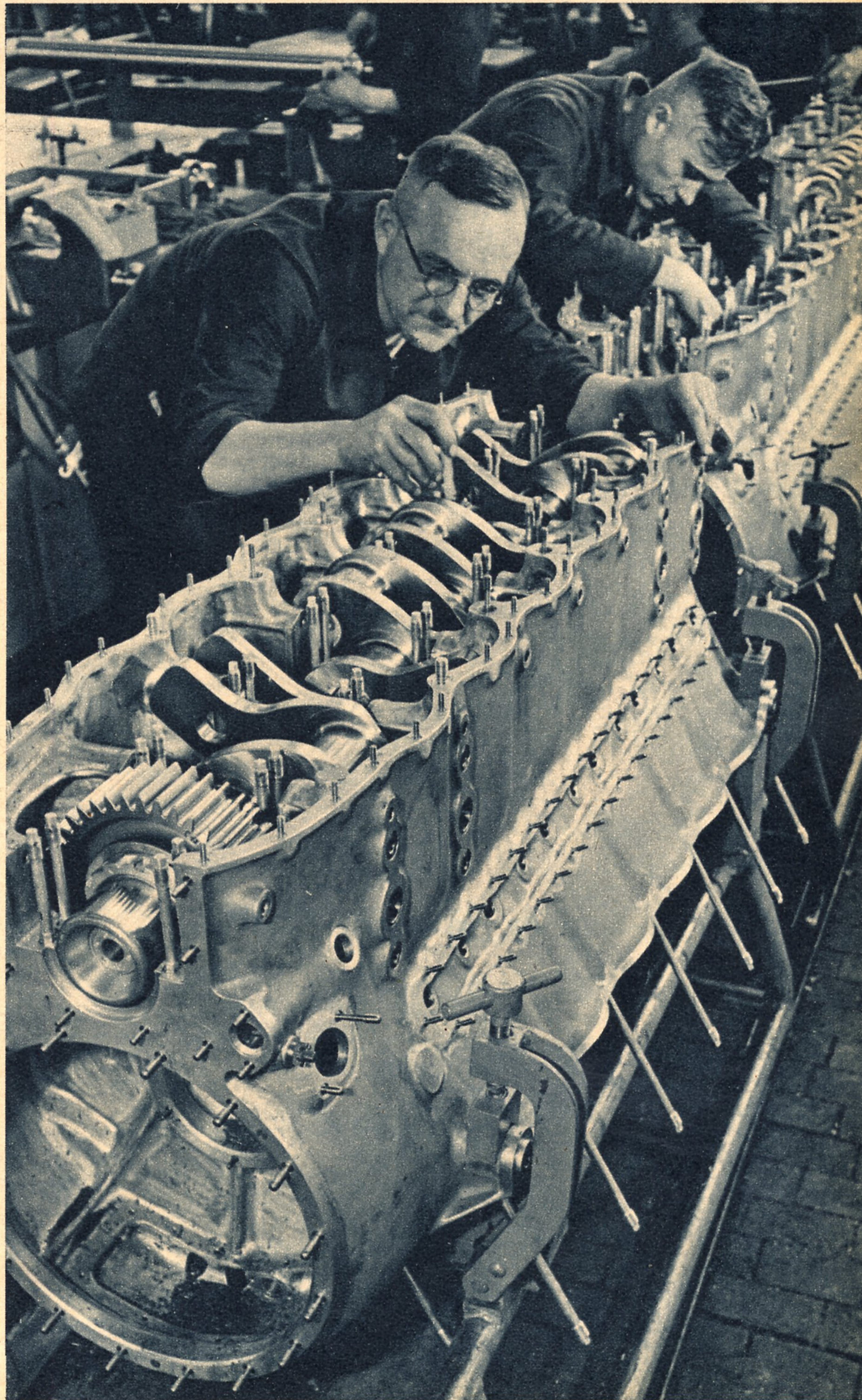
Zum Bilde rechts: Flugzeugmotoren, die über viele PS verfügen, im Serienbau. Die Facharbeiter sind gerade mit dem Einbau der Kurbelwelle beschäftigt. Aufn. J.F.N.
