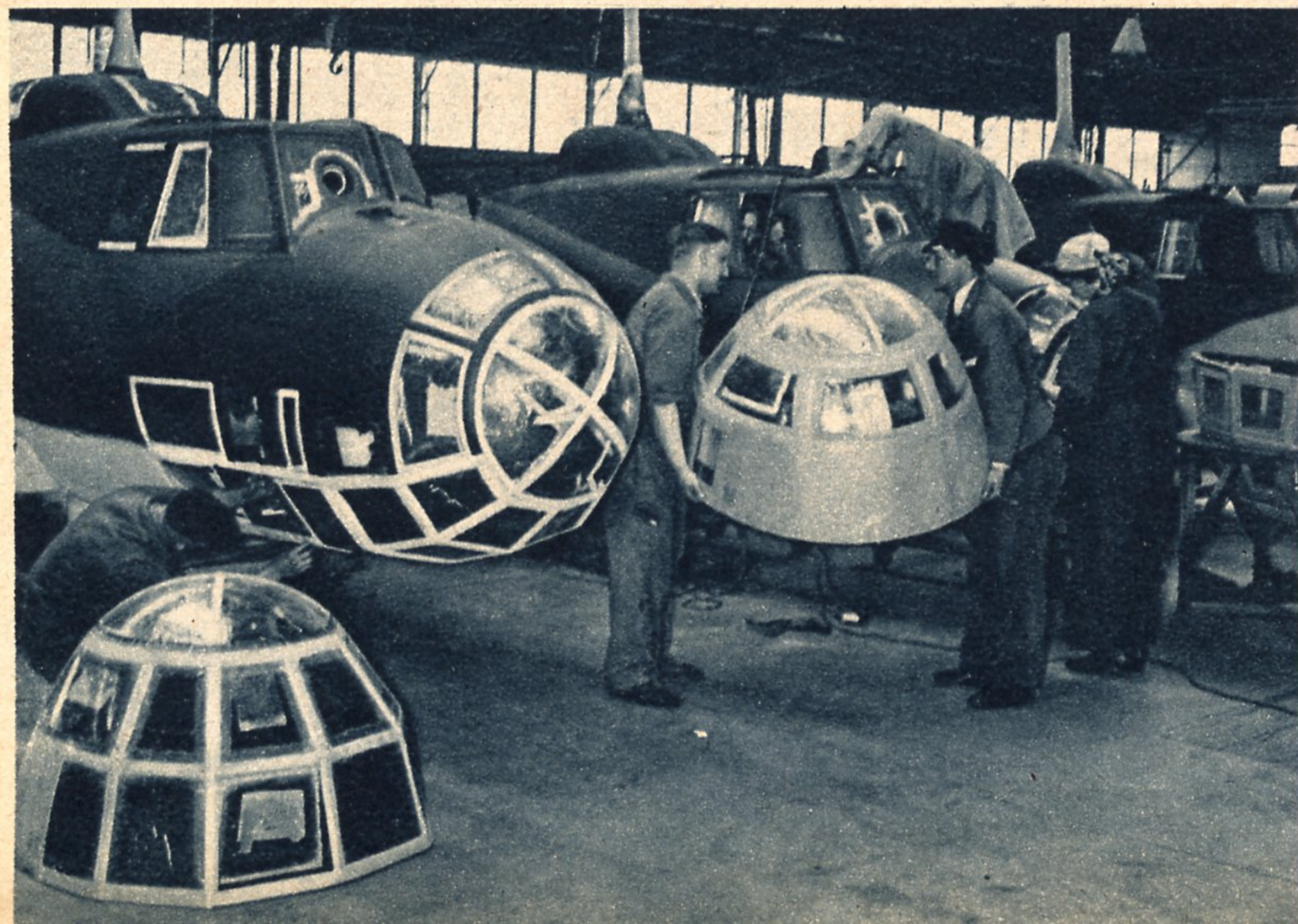
Unten: Einbau der aus durchsichtigem Werkstoff hergestellten Kanzeln in die Kampfflugzeuge Aufn. Stöcker (2)
